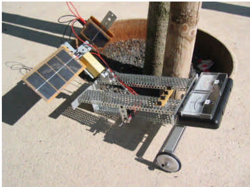
Nachgeführtes Solarpanel
